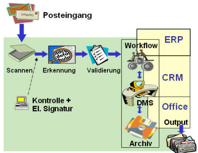
Abbildung 2 : Elektronische Posteingangsbearbeitung
